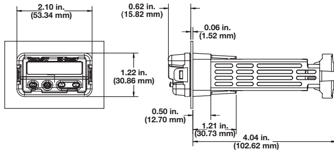
EZ-ZONE PM 1/2 DIN
