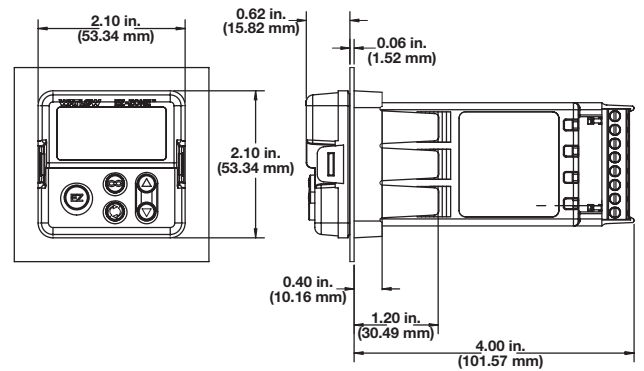
EZ-ZONE PM 1/6 DIN
